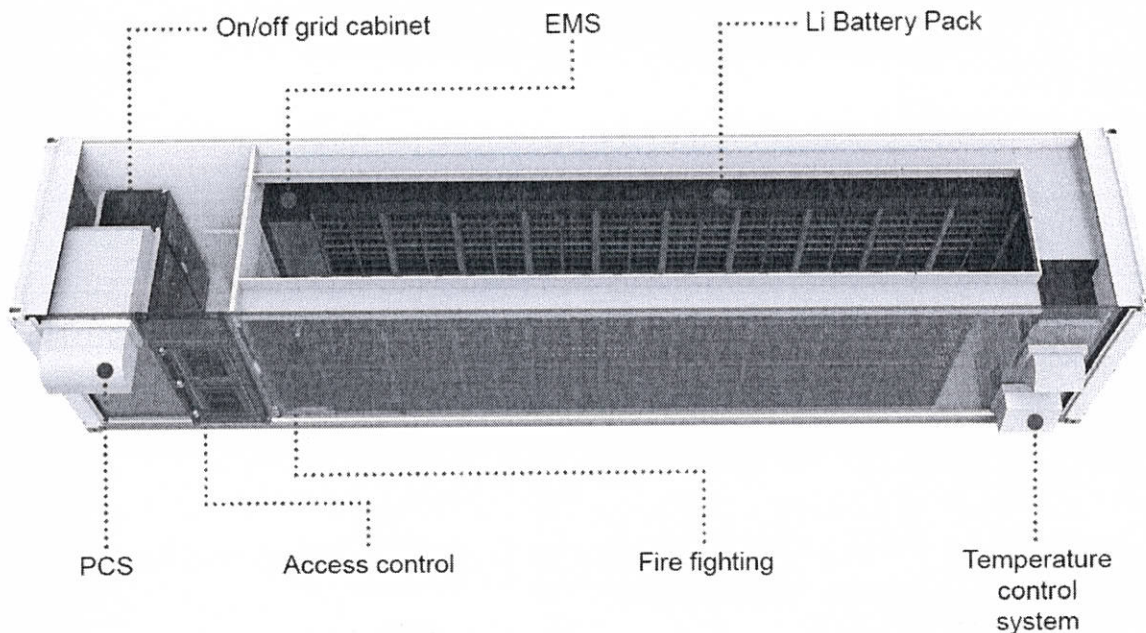
Εικόνα 1: Τυπική διάταξη συστήματος αποθήκευσης ενέργειας επί Container
