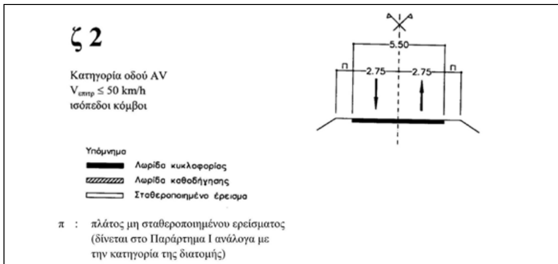
Διάγραμμα 1: Τυπική Διατομή
